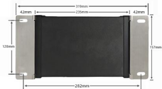
安装尺寸图
